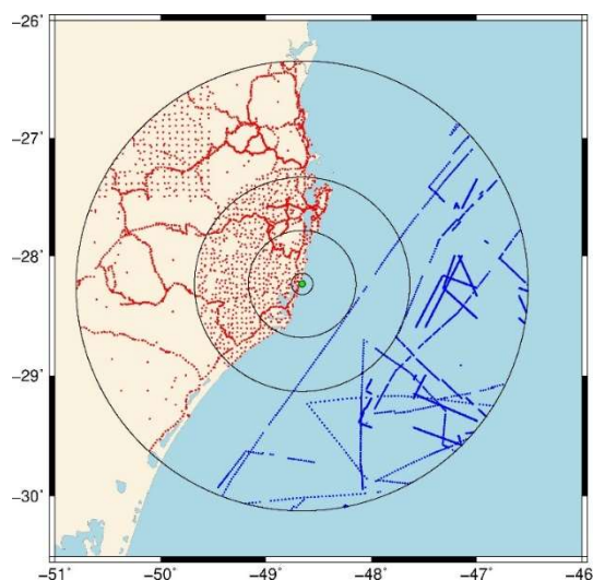
Figura 2 – Distribuição de medidas gravimétricas terrestre (em vermelho) e marinha (em azul) na estação IMBT, Brasil.
